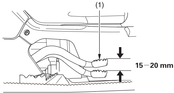
(1) takajarrupoljin
