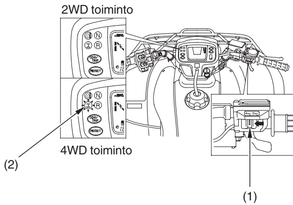
(1) 2WD/4WD valintakytkin
