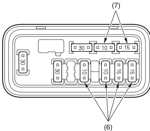
(6) käyttösulakkeet
