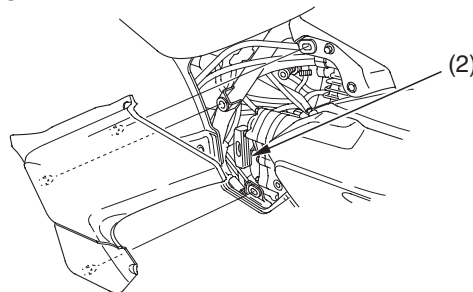
(2) käsi käynnistin
